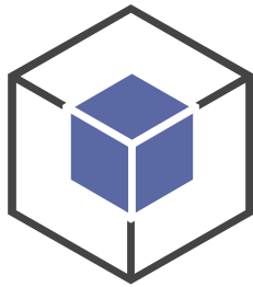
PHP server
