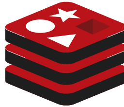
Redis
