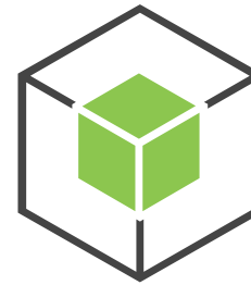
Node.js
